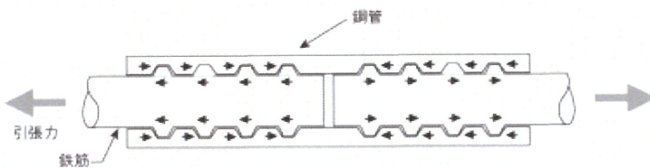
機械式継手の原理
